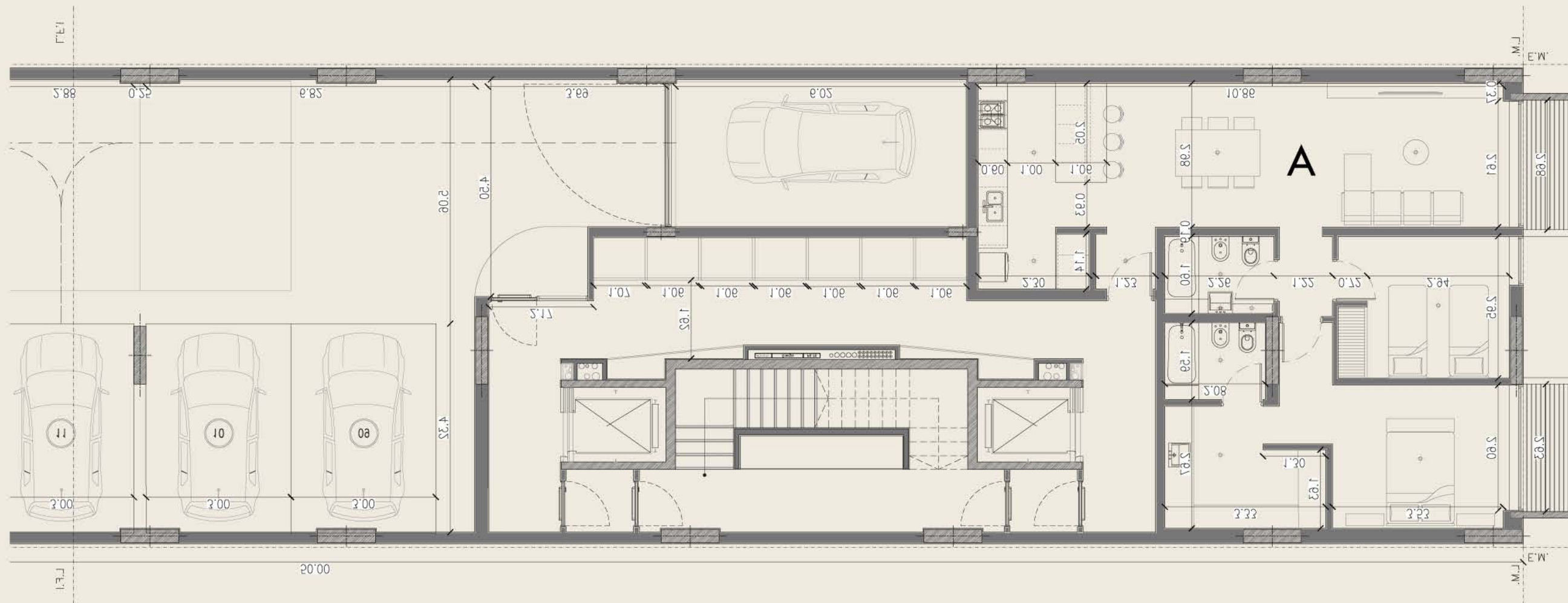
NIVEL 1 - COCHERAS Y VIVIENDA 2 DORMITORIOS
